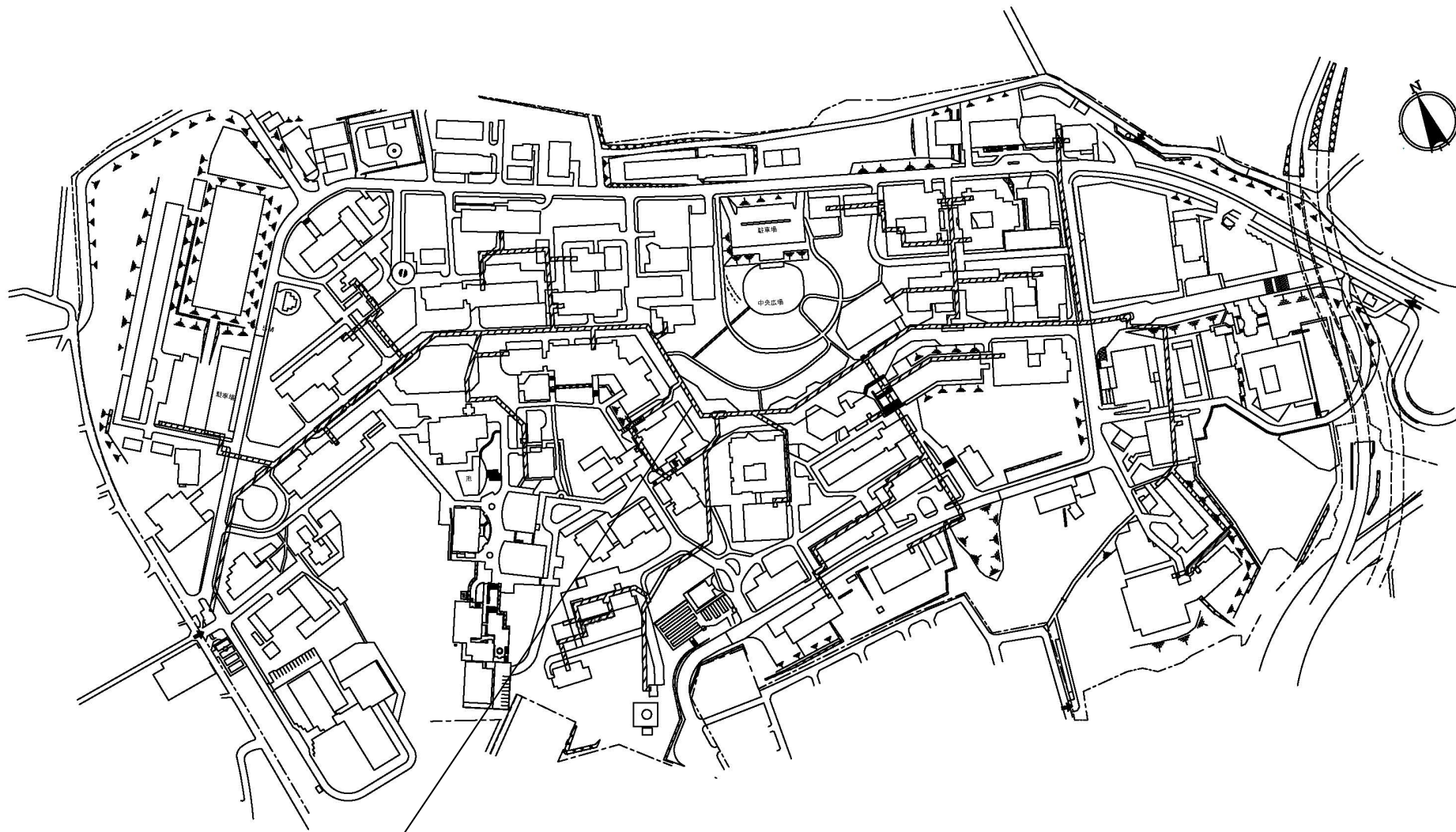
屋内消火栓用屋外配管の更新範囲
