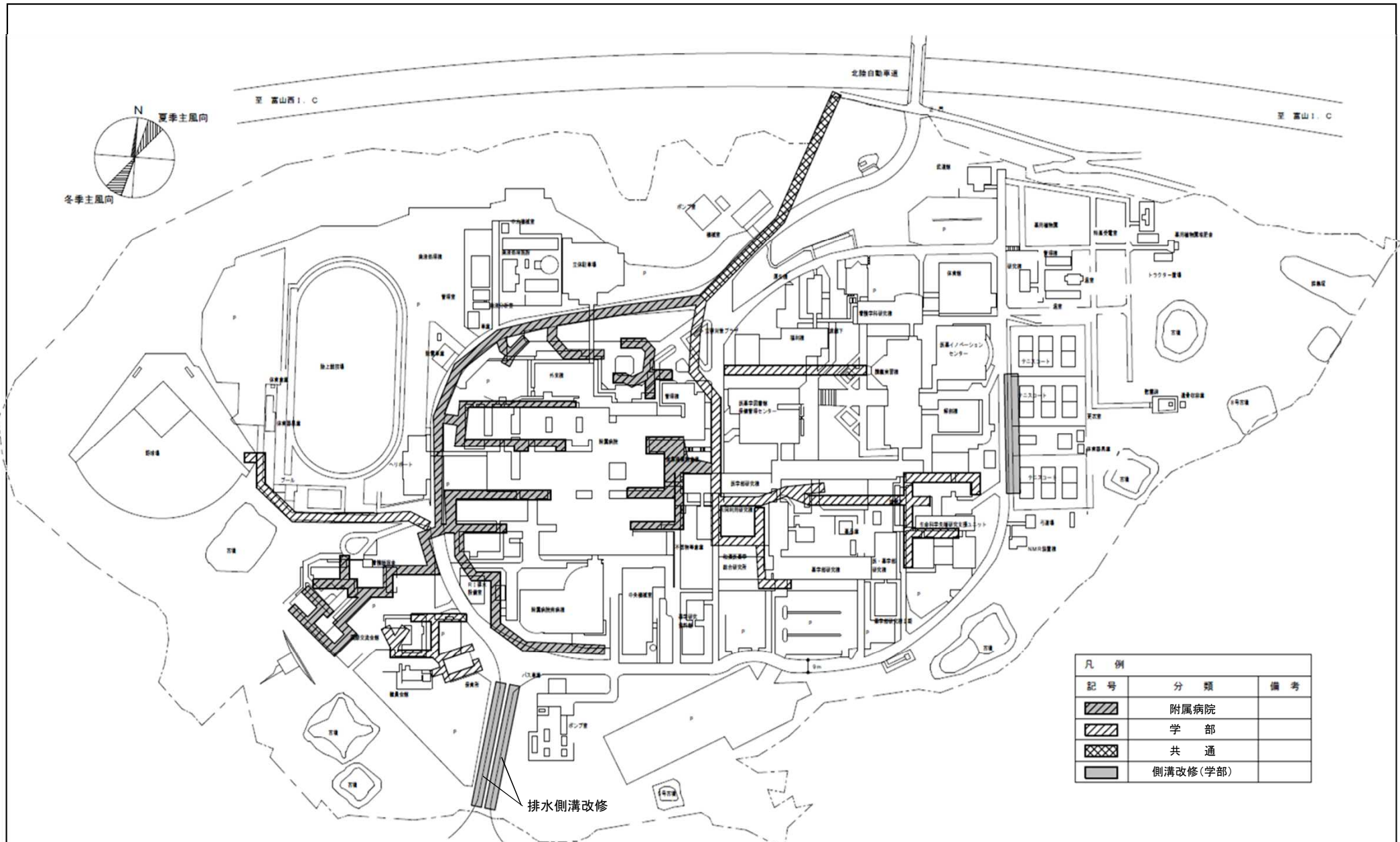
雨水排水管配置図
